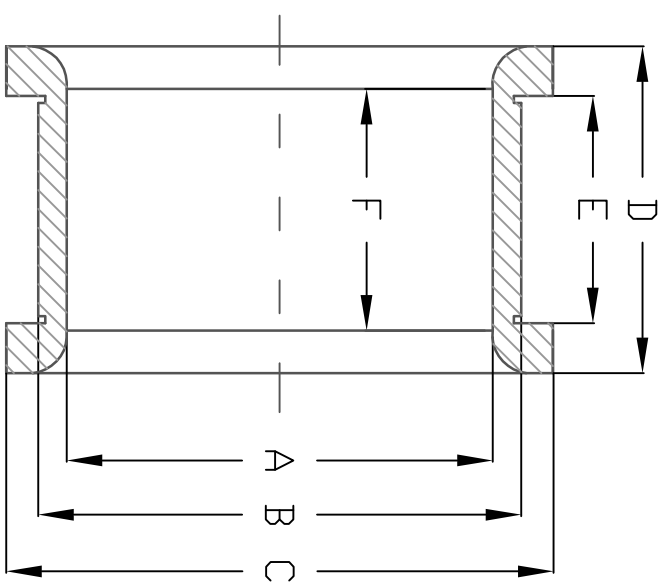
Schnitt A-A
